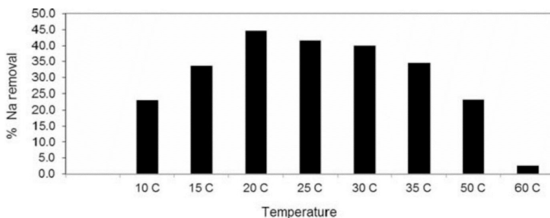
Figuur 5 Verwijderingsefficiëntie van natrium uit Produced Water bij verschillende temperaturen (Chaalal et al, 2015)
