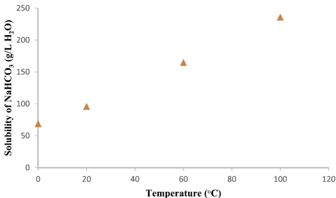
Figuur 4: Oplosbaarheid van natriumbicarbonaat in water bij verschillende temperaturen [36]
